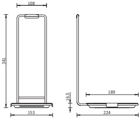
Schalenhalter mit Bügel und Schale 1000
