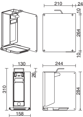
Montagewinkel 500 (links)
