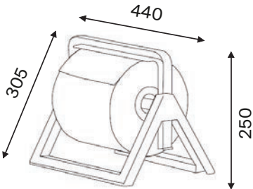
Wandmodell
