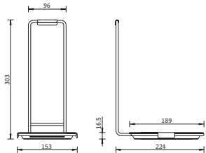
Schalenhalter mit Bügel und Schale 500
