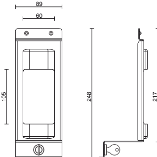
Verschlussblende für V/VK-P-Spender 1000
