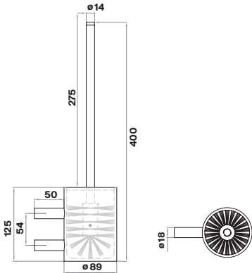
WC-Bürste rund
