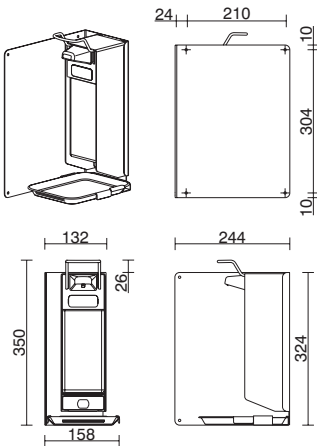
Montagewinkel 1000 (rechts)
