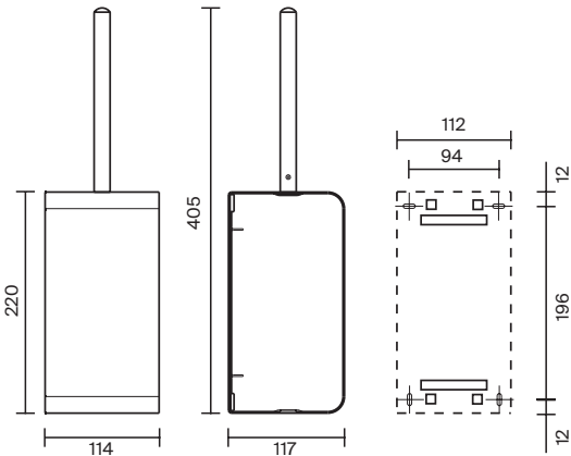
WC-Bürste
