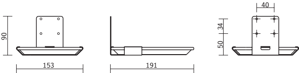
Tropfschale Unterbau
