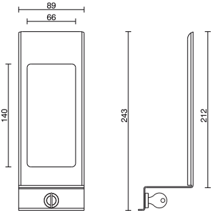
Verschlussblende E-Spender 1000
